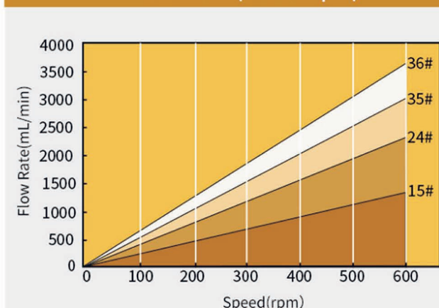
Flow Rate(0.1-600rpm)
